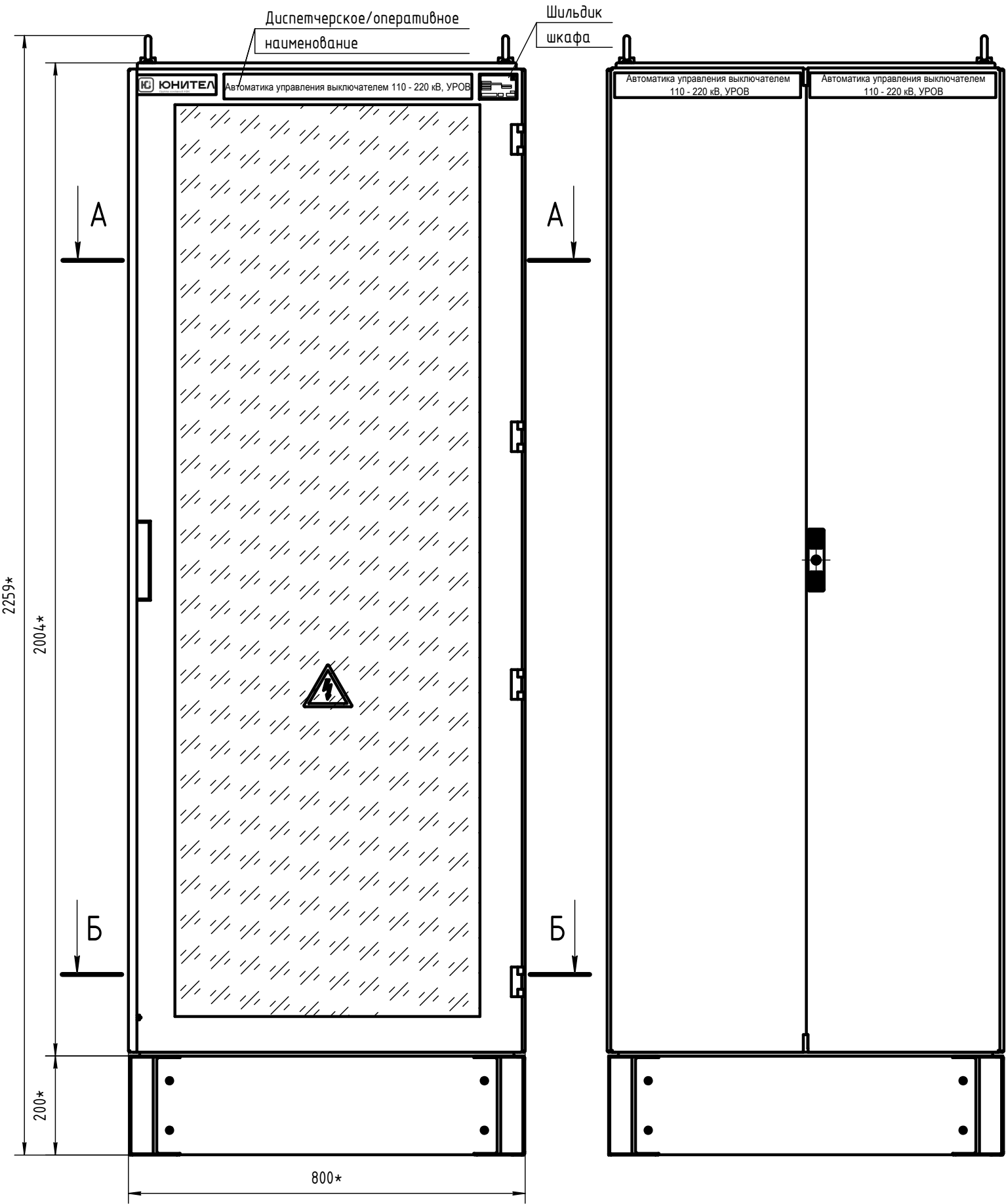
Вид сзади
